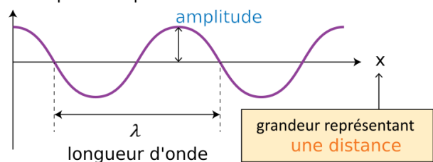
champ électrique en à un instant donné
