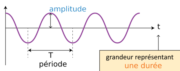
champ électrique en un point du milieu
